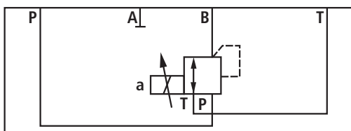
类型 3DREP..6 B 2X/..E (详细)
