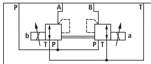
带集成控制电子元件的阀示例 类型 3DREPE..6 C 2X/..E (简化)
