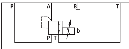
类型 3DREP..6 A 2X/..E (详细)
