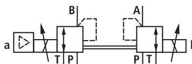
带集成控制电子元件的阀示例 类型 3DREPE..6 C 2X/..E (简化)
